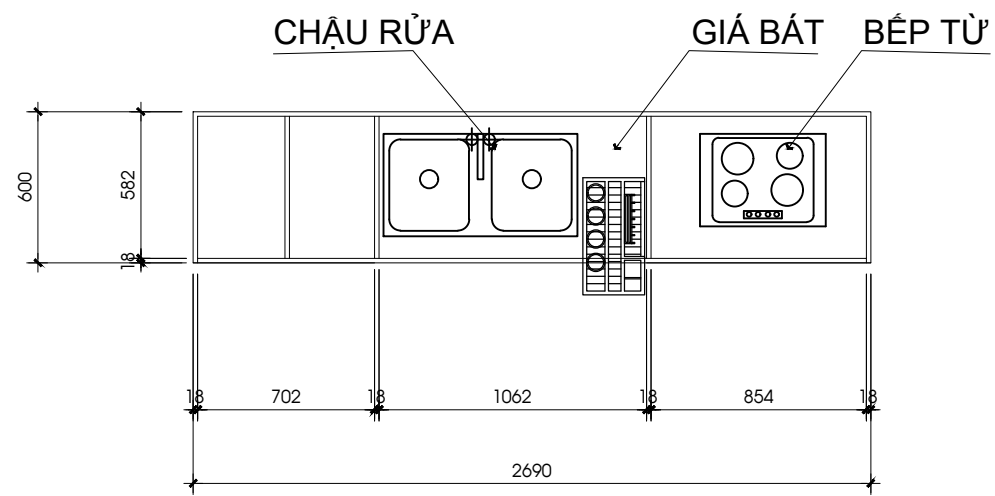
MẶT BẰNG TỦ DƯỚI
